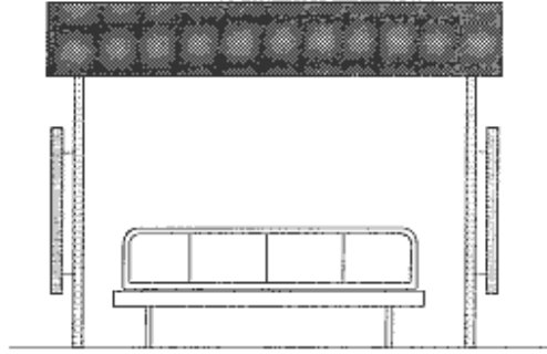
واجهة للمحطة
